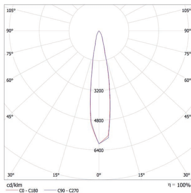
reflektor 15°
