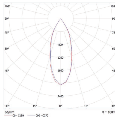
reflektor 35°
